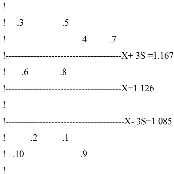
Fig. 3.3 Gráfico de control para la determinación de las zonas de laterita de balance.
