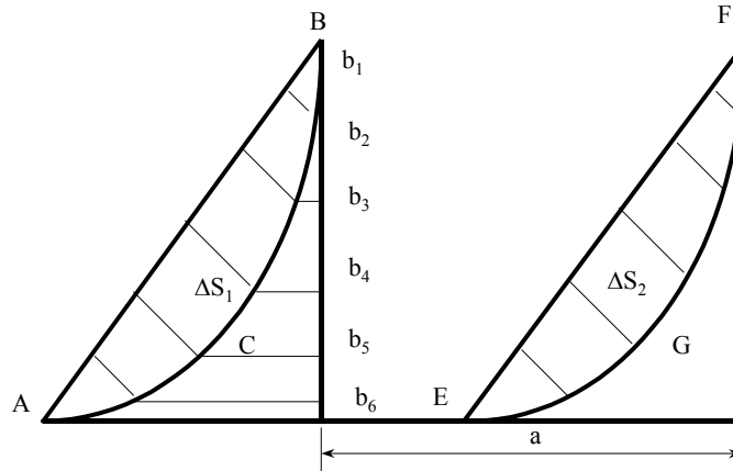
Fig.2.4 Configuración de los perfiles del talud.
