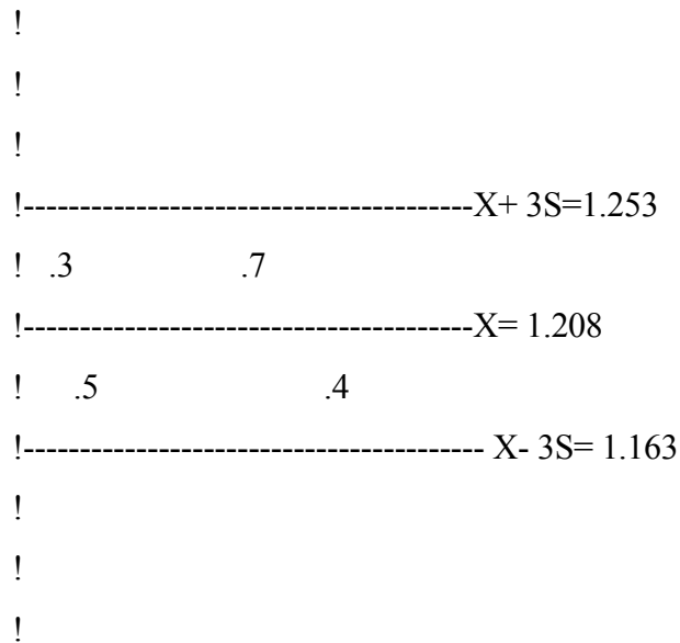
Fig. 3.4 Gráfico de control para la determinación de las zonas de serpentina blanda.
